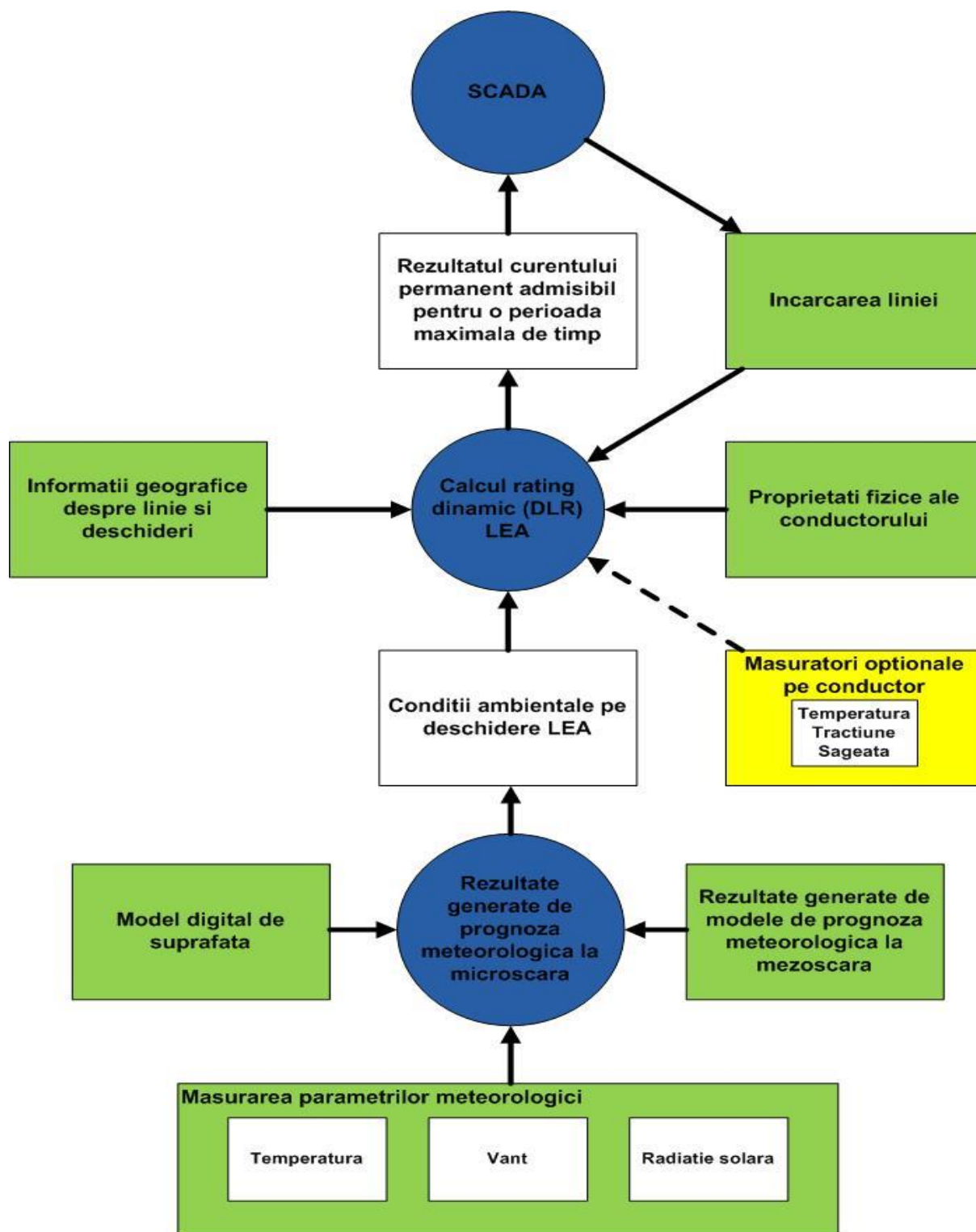
Figura 3: Implementarea posibilă a diferitelor surse de date meteorologice pentru calculul curentului permanent admisibil
